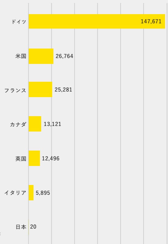
各国の難民認定数(2017年) [単位]人
